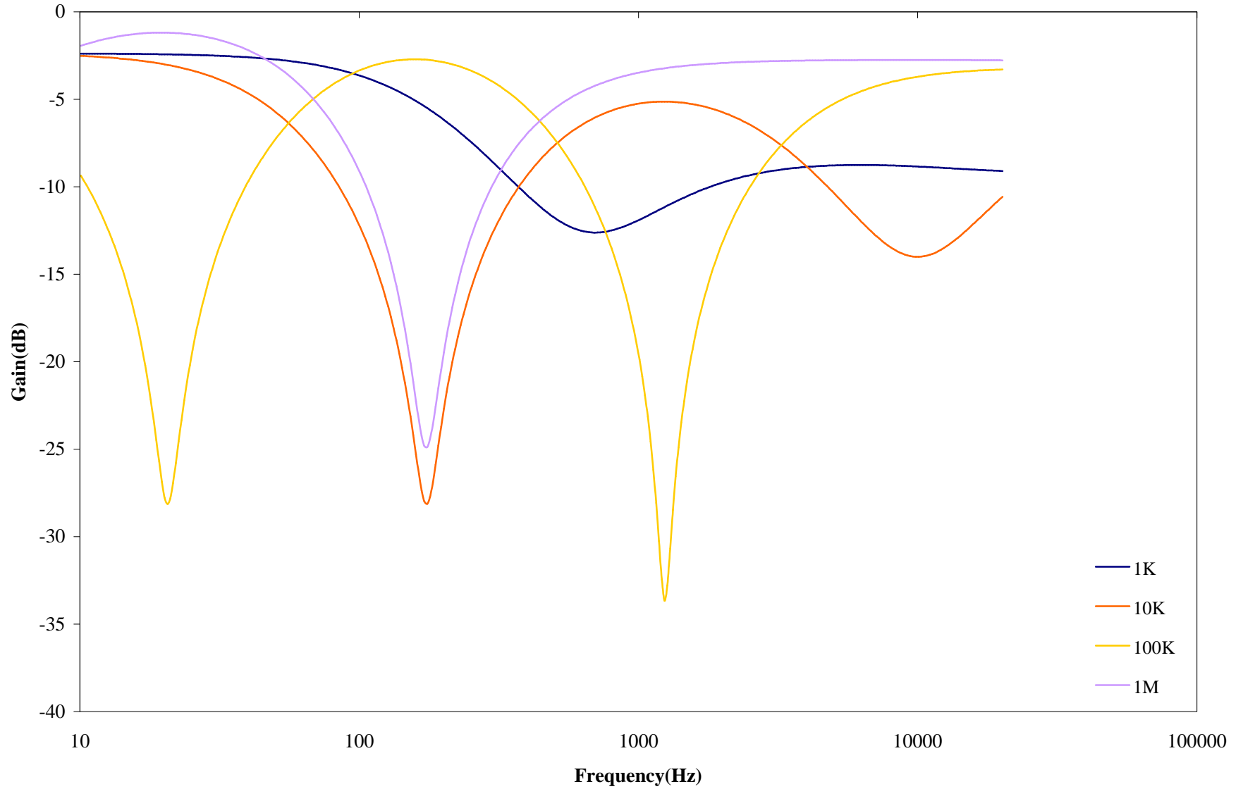
Uni-Vibe - 22nF, 220nF, 470pF & 4.7nF
